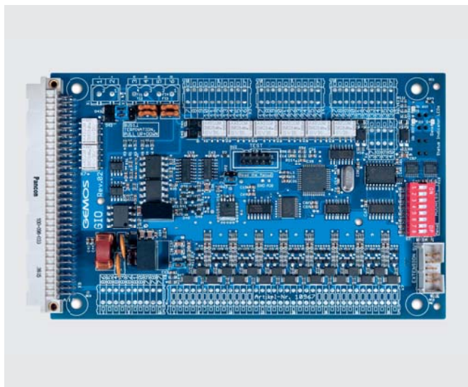
GEMOS input output module GIO-VG
