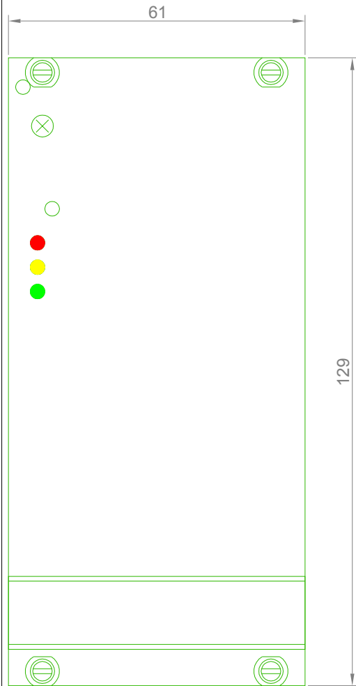
Netzteil Frontansicht
