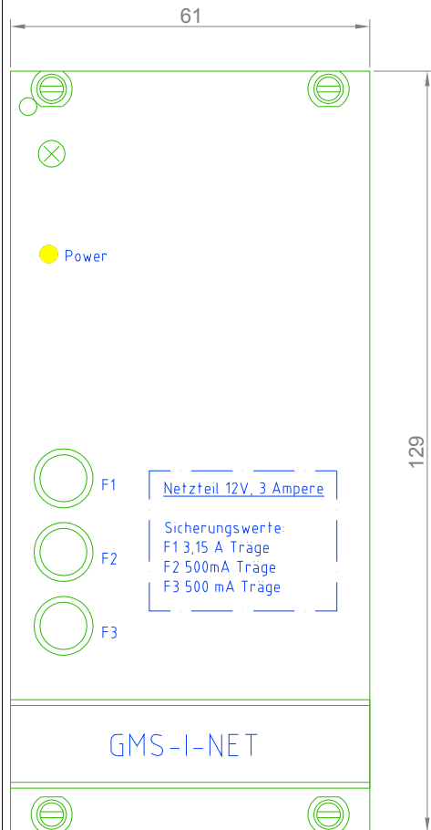
Netzteil Frontansicht
