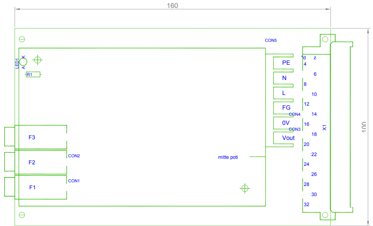
Netzteil Seitenansicht
