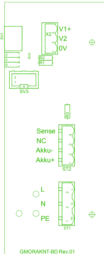
Rückwandplatine im 19" Rack
